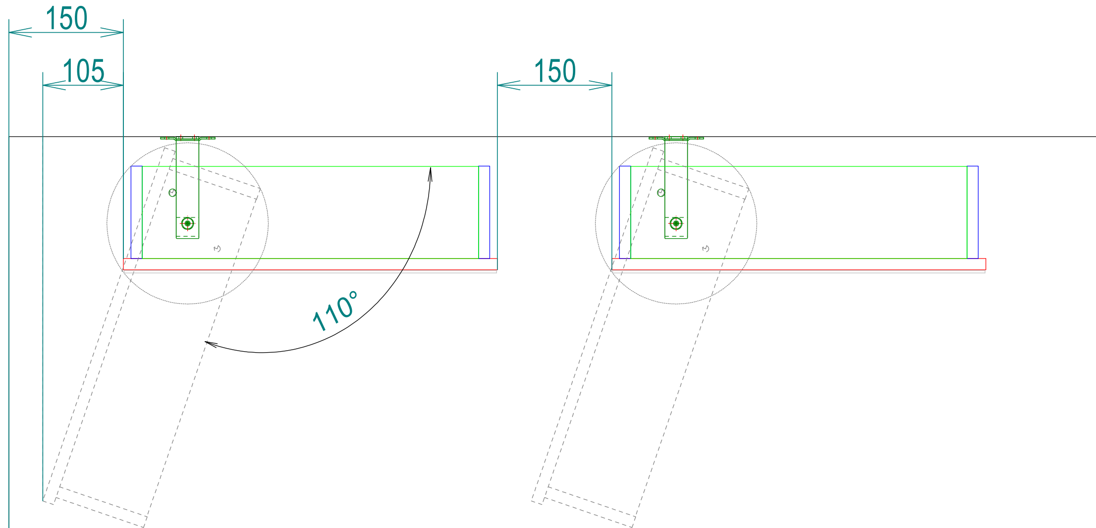
Abstände Mehrzweckdrehschrank 1186; 1189; 1195 und 1196
